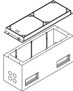
P-Schacht V-A - 174/68 (als Aufbauschacht, längsgeteilt)
