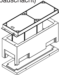
P-Schacht IV-A - 160/50/70 (als Aufbauschacht)
