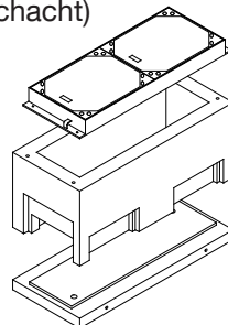
P-Schacht VI-A - 120/40/60 (als Aufbauschacht)
