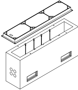
P-Schacht II-A - 160/40/70 (als Aufbauschacht)
