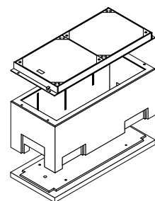
P-Schacht V-A - 174/68 (als Aufbauschacht, längsgeteilt)
