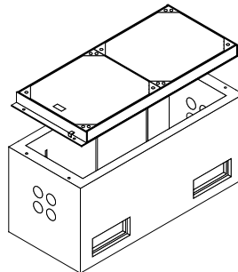
P-Schacht VI-A - 120/40/60 (als Aufbauschacht)
