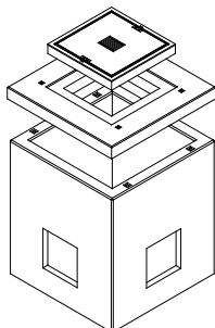
Topfschacht 120/120/150
