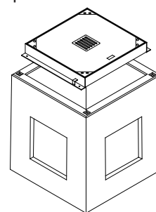
Topfschacht 100/100/100
