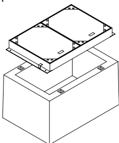
Topfschacht 100/100/150
