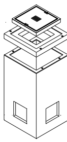
Topfschacht 125/95/134
