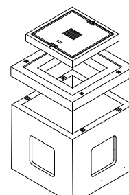
Topfschacht 120/120/100
