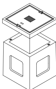
Topfschacht 100/80/100
