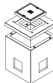
Topfschacht 120/120/100
