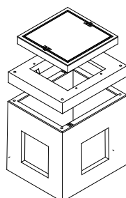
Topfschacht 100/100/200
