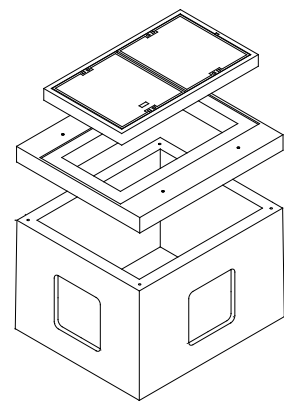
Topfschacht 150/150/100
