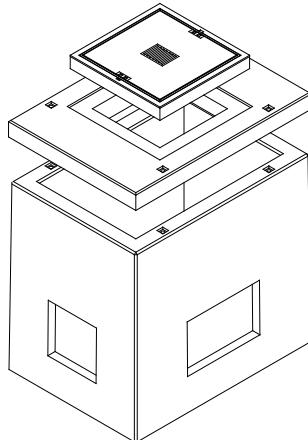
Topfschacht 150/100/150
