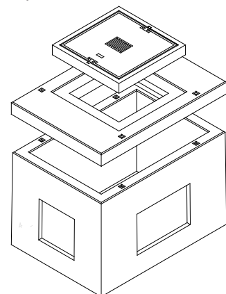
Topfschacht 200/150/100
