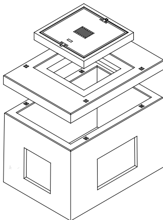
Topfschacht 150/100/100
