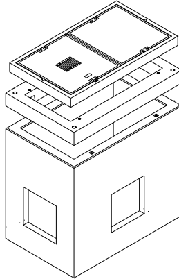
Topfschacht 150/100/150
