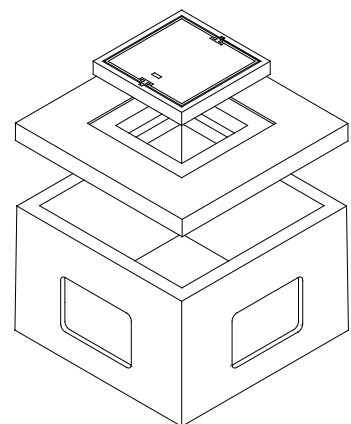
Topfschacht 150/150/100
