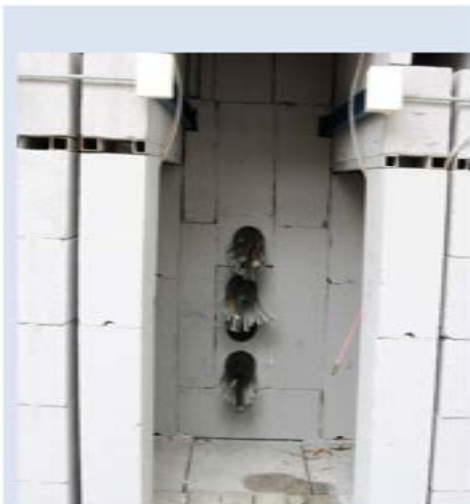
Prüfkonstruktion für Kabel- und Fugen-Abdichtung
